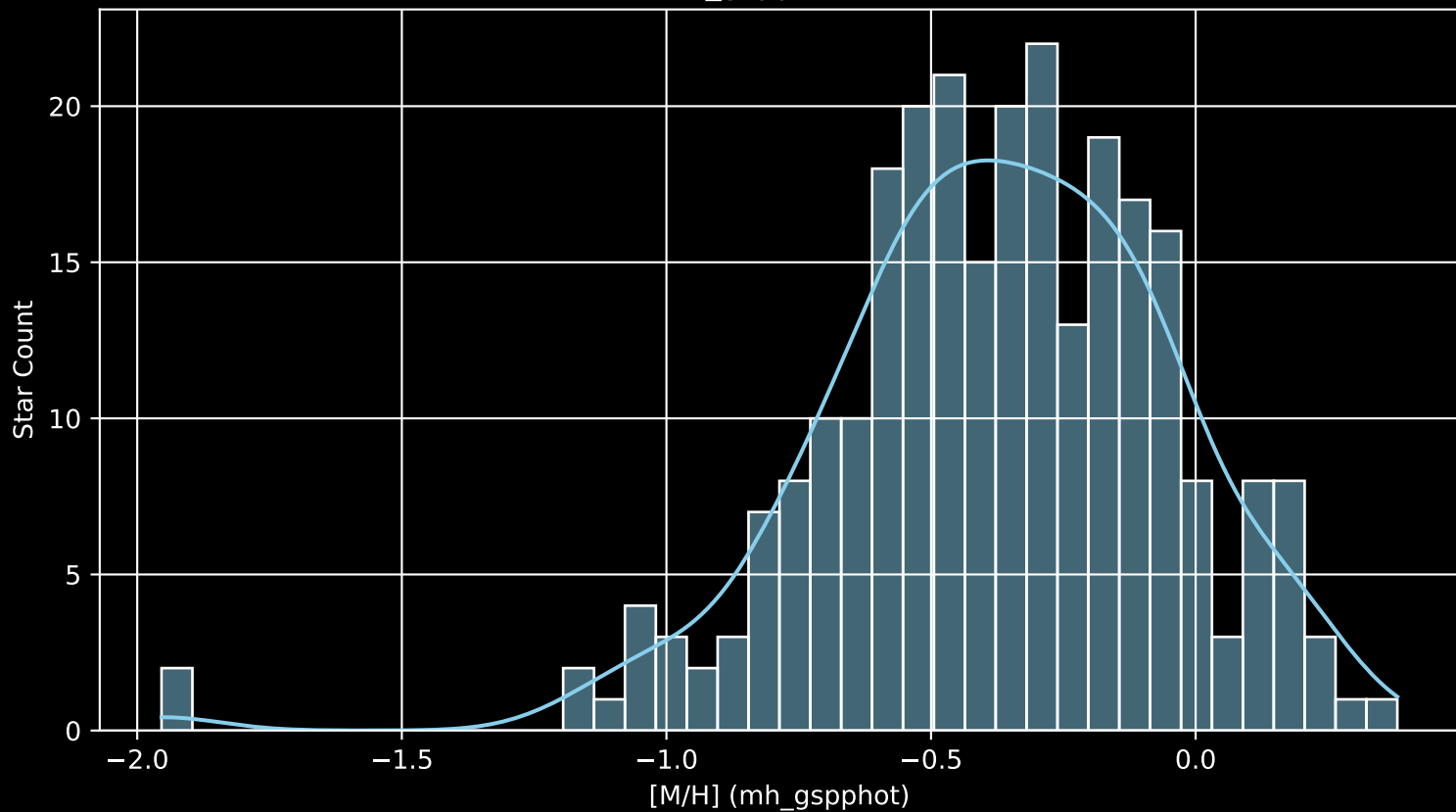
GALAH DR4 Field: [542] [M/H] (mh_gspphot) (n= 265)
