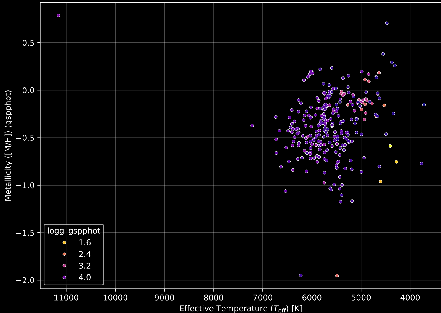
GALAH DR4 Field: [542] Stellar Population Parameters (n= 267)
